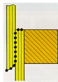
Figuur I Goed uitgevoerde horizontale naad met overlapafschuining en 'gebroken' kant.
